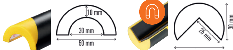
art. 1115 - Profilo paracolpi per tubolari P30
