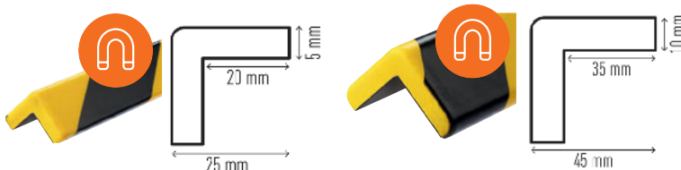
art. 1111 - Profilo paracolpi angolare C20
